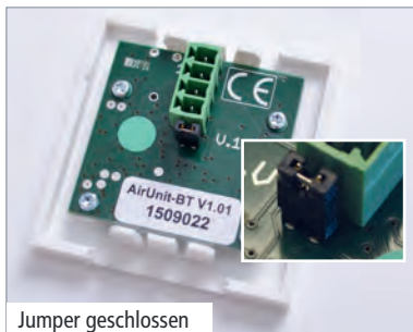
Jumper geschlossen
