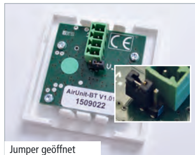
Jumper geöffnet
