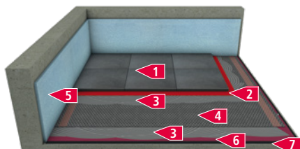
Fußbodenheizung (verklebt)
