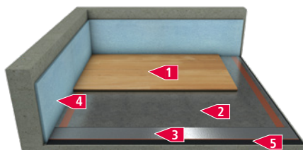
Fußbodenheizung (schwimmend)
