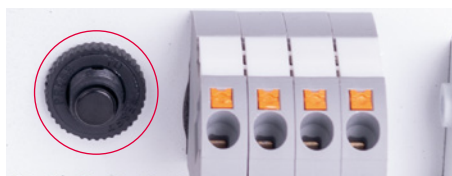
Heizkreissicherung durch Drücken zurücksetzen
