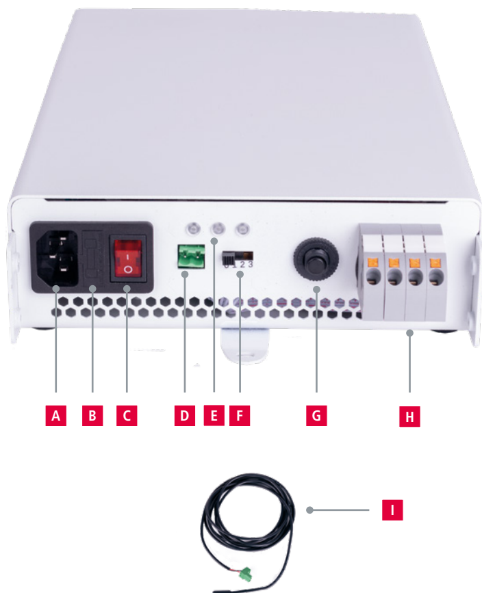
HF Netzteil SelfTec 300 W (ohne untere Abdeckung)
